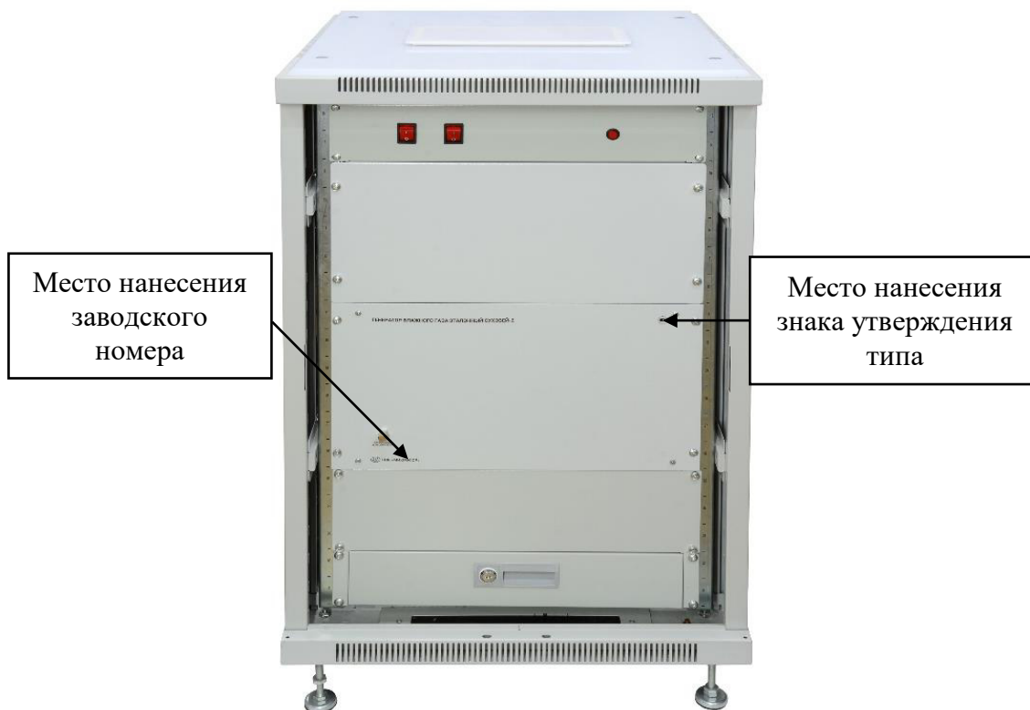
Рисунок 2 - Внешний вид генератора влажного газа эталонного Суховой-2 с указанием мест нанесения знака утверждения типа и заводского номера.
