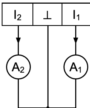
Рис.4. Подключение вторичных приборов к токовым выходам.
