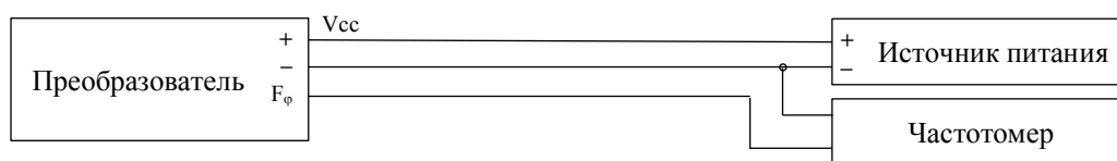
Рисунок 1 – Схема подключения преобразователя исполнения ДВ2М (с частотным выходом).
