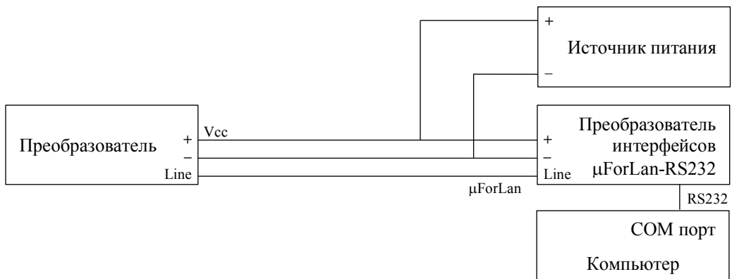
Рисунок 6 – Схема подключения преобразователя исполнения ДВ2ТСМ 4П и АК (с интерфейсом \mu ForLan).
