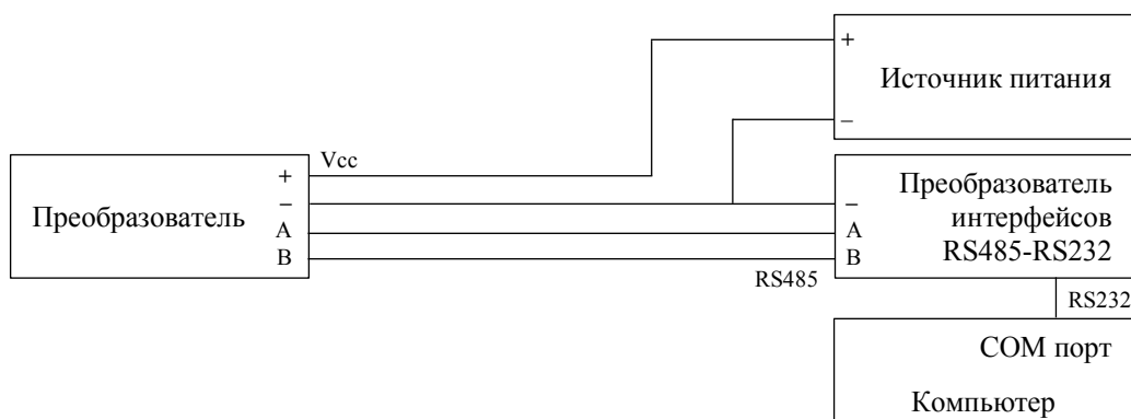
Рисунок 4 – Схема подключения преобразователя исполнения ДВ2ТС (с выходным интерфейсом RS485).
