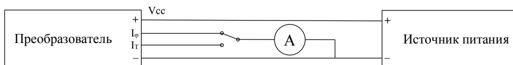
Рисунок 3 – Схема подключения преобразователя исполнений ТТ20-А и ТТ20-Г (с токовыми выходами 4...20мА).
